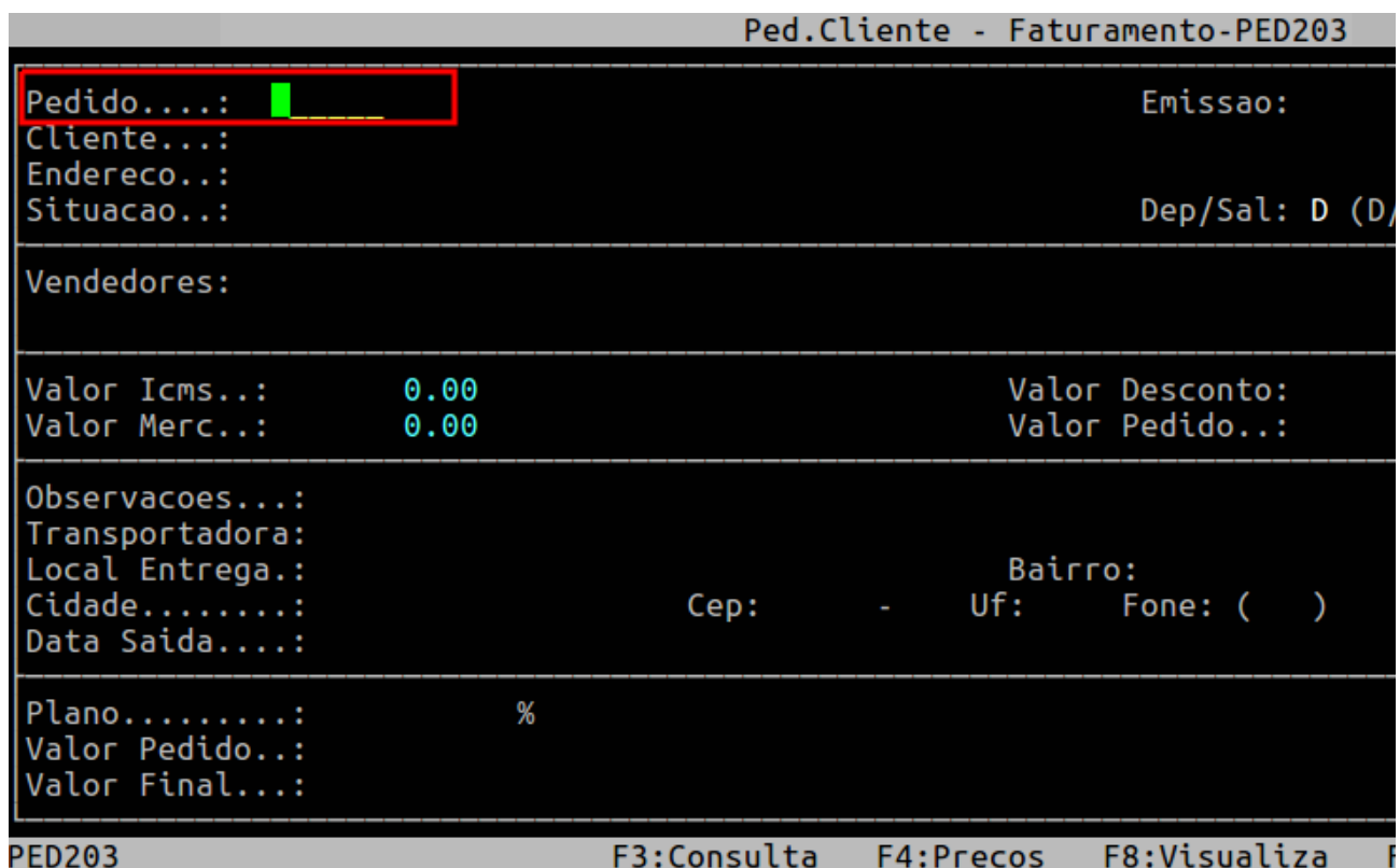
Exemplo da Tela de Faturamento de Pedido de Cliente - Informando o Número do Pedido
